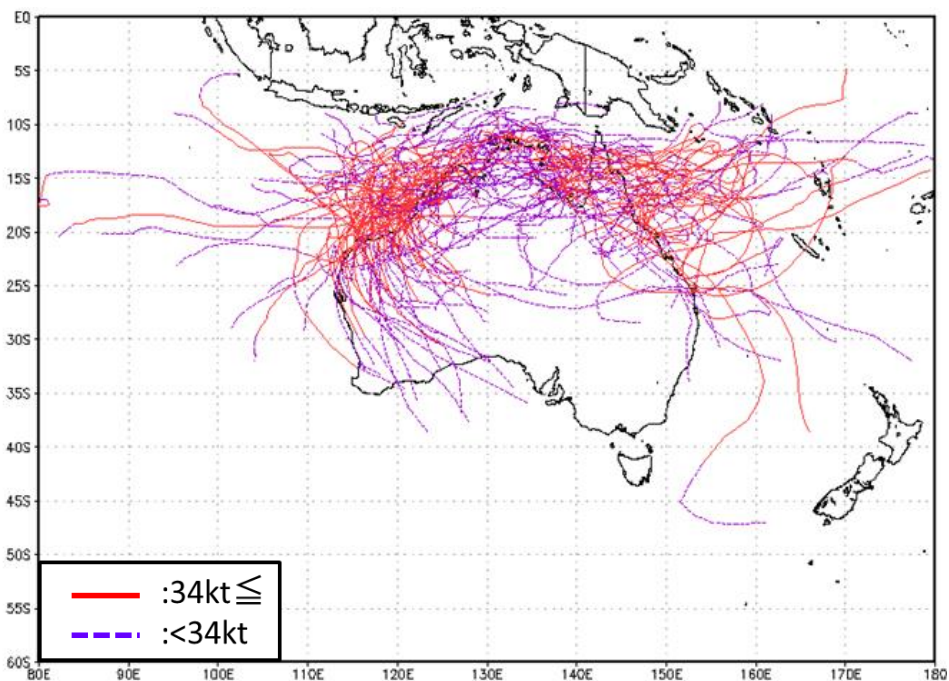
図 4.26 オーストラリアに上陸する台風経路図(2001-2011)
