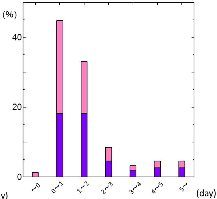
図 4.33 台風上陸から消滅までの日数別頻度図(1970-2011)
