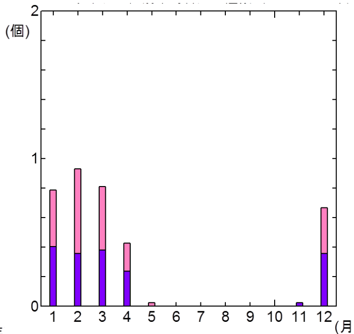
図 4.28 オーストラリアの月別平均台風上陸数(2001-2011)
