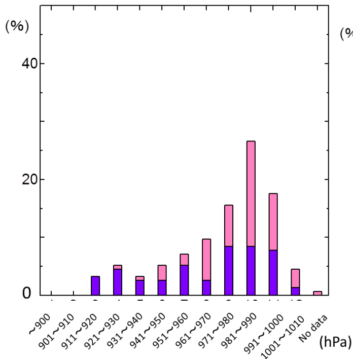
図 4.30 上陸時の気圧別頻度図(1970-2011)
