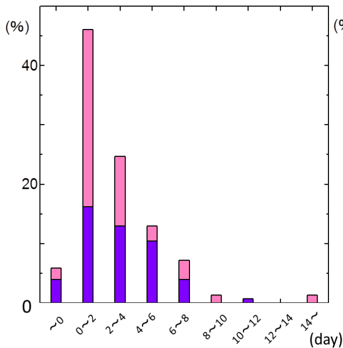
図 4.32 台風発生から上陸までの日数別頻度図(1970-2011)
