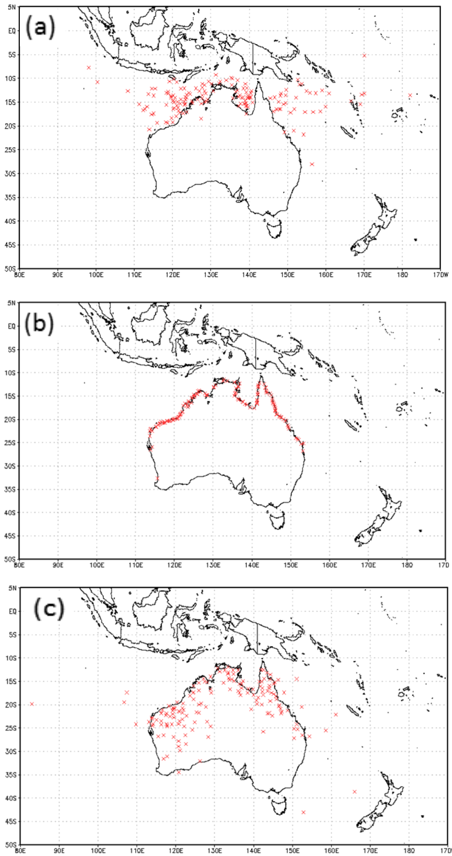
図 4.29 オーストラリアに上陸する台風の(a)発生(b)上陸(c)消滅地点(2001-2011)
