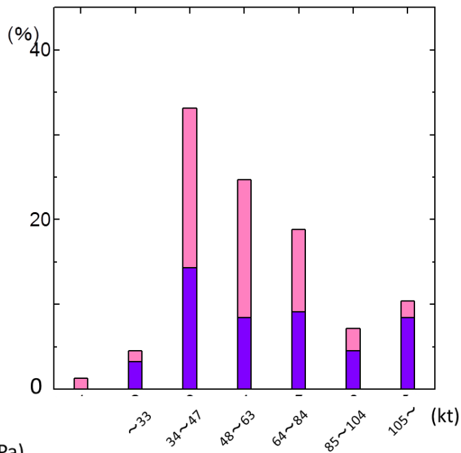
図 4.31 上陸時の風速別頻度図(1970-2011)
