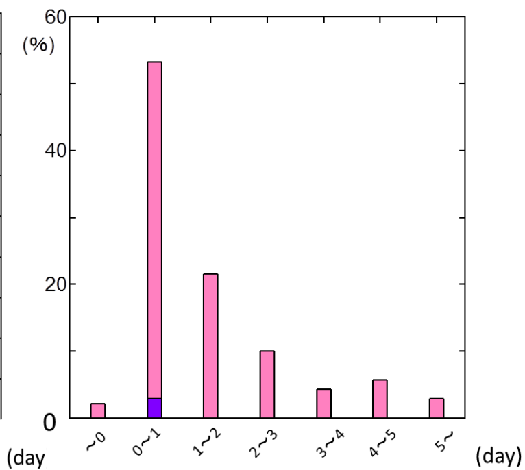
図 4.41 台風上陸から消滅までの日数別頻度図(1970-2011)
