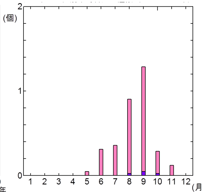
図 4.36 アメリカの月別平均 台風上陸数(2001-2011)
