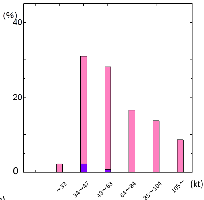
図 4.39 上陸時の風速別頻度図(1970-2011)
