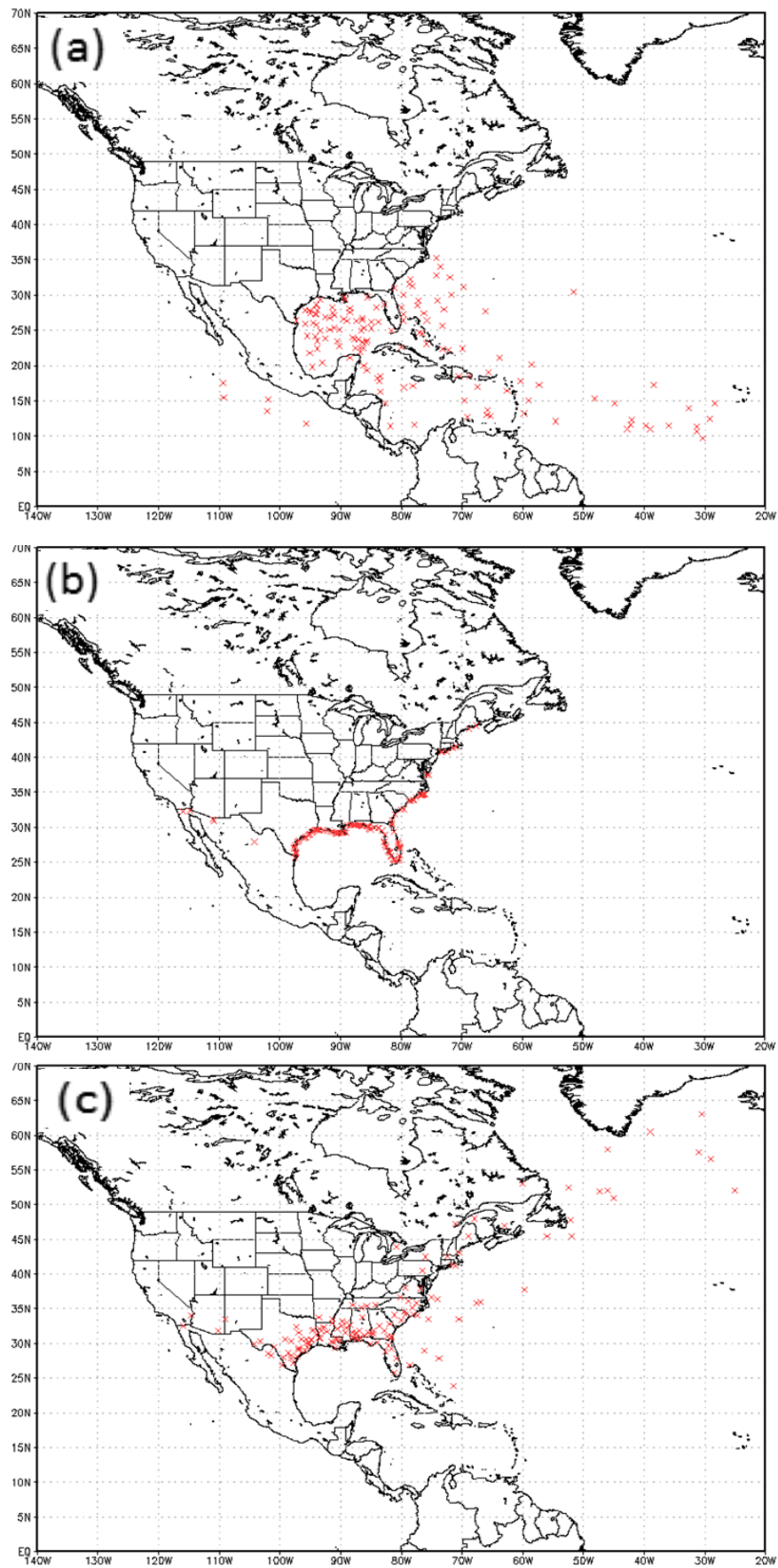
図 4.37 アメリカに上陸する台風の(a)発生(b)上陸(c)消滅地点(2001-2011)
