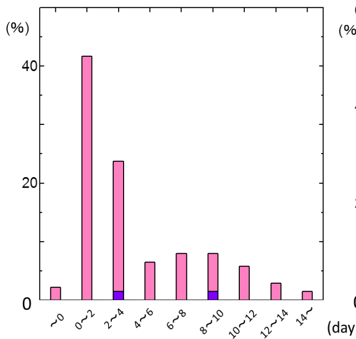
図 4.40 台風発生から上陸までの日数別頻度図(1970-2011)
