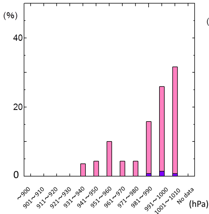
図 4.38 上陸時の気圧別頻度図(1970-2011)
