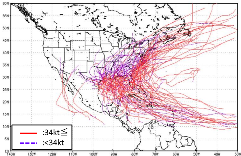
図 4.34 アメリカに上陸する台風経路図(2001-2011)
